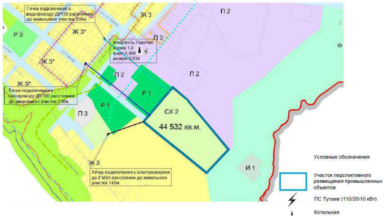
Схема участка №5 (76:21:000000:231)
